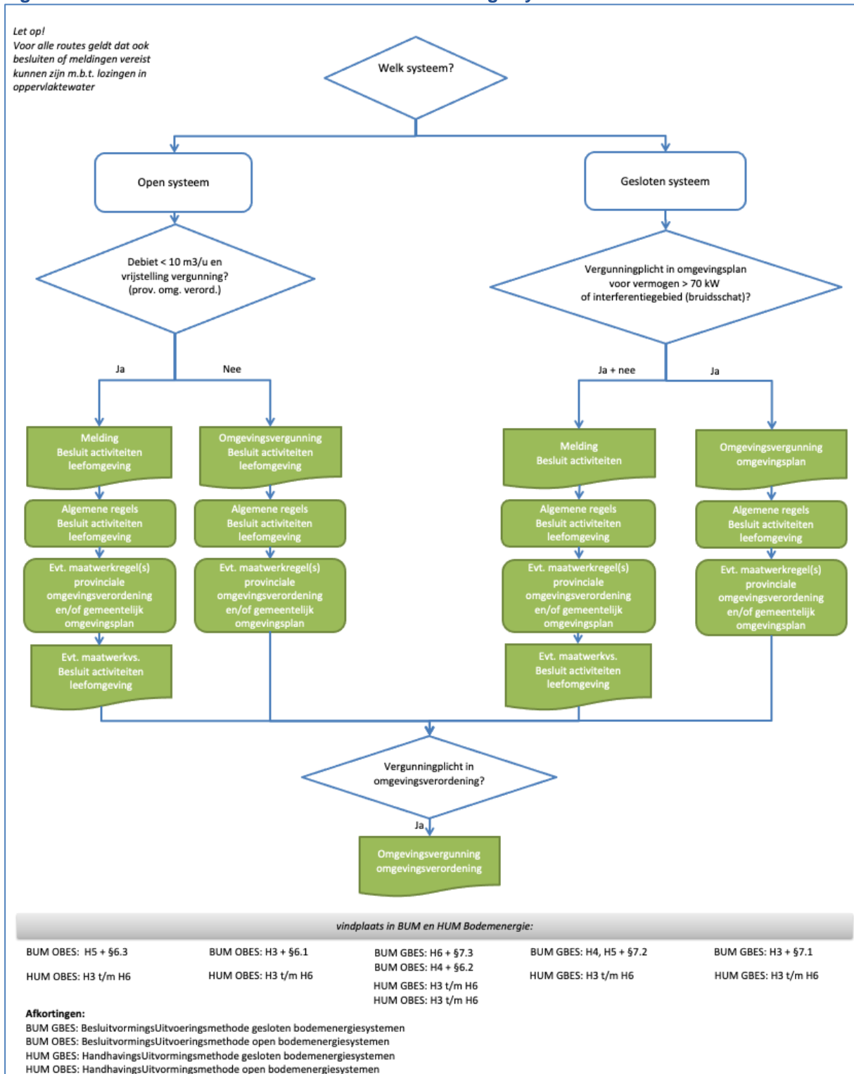
Figuur 1.3. Stroomschema besluiten m.b.t. bodemengiesystemen.
