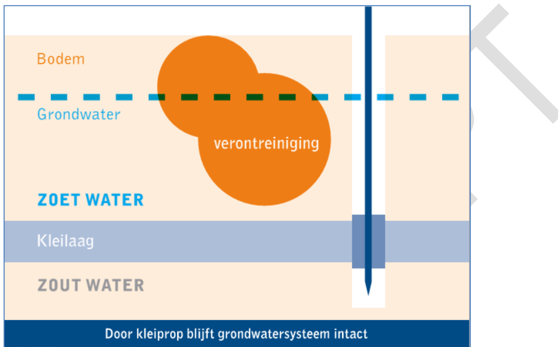
Figuur 4.1. Illustratie voorkomen vermenging van grondwater met verschillende kwaliteiten
