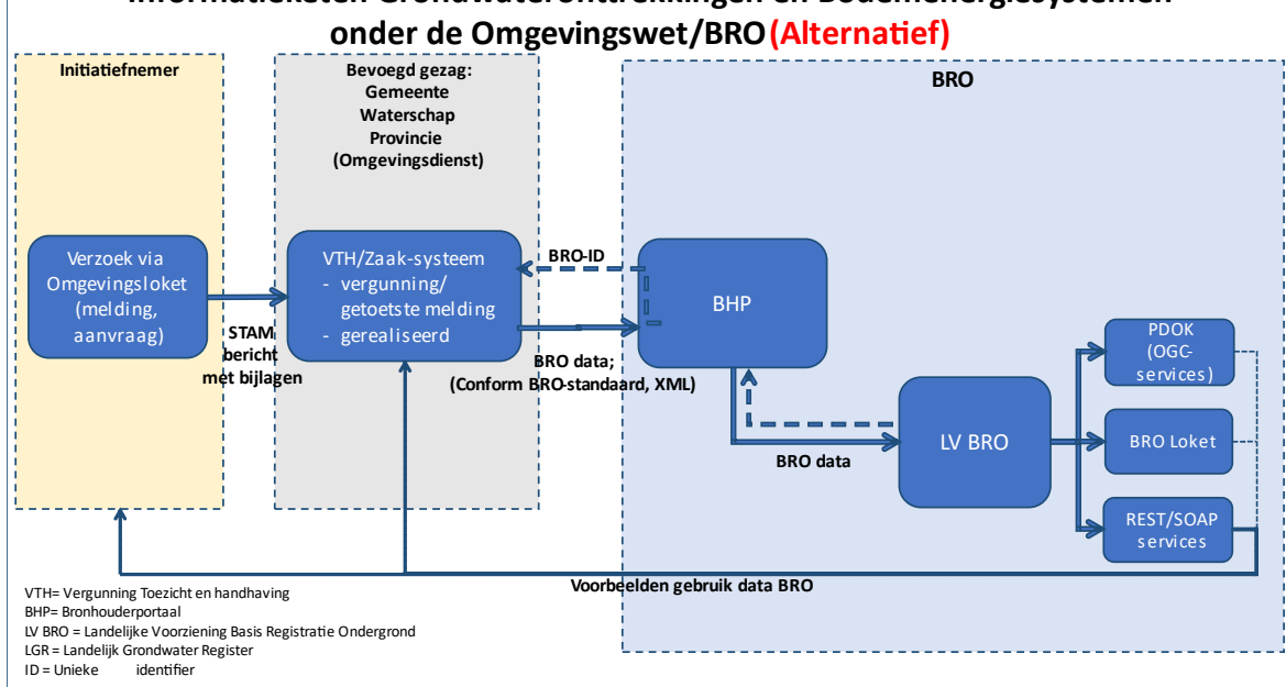
Figuur 6.2 Alternatieve informatieketen gegevens bodemenergiesystemen per 1 juli 2022 Informatieketen Grondwateronttrekkingen en Bodemenergiesystemen
